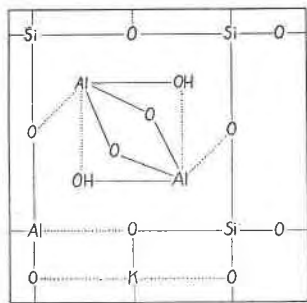
( ^2 OH) _2 K _1 Al _2 ( ^1 Si _3 Al) _1 O _{10}
