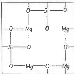
FIG. 7. Forsterite.
