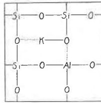
FIG. 20. Orthoclase.
