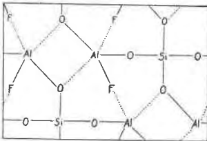
FIG. 12. Topaz.
