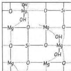
FIG. 8. Norbergite.
