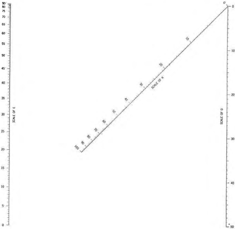
PLATE IV. NOMOGRAM OF D · K · SIN E (Mallard's formula) JOHN B. MERTIE, JR. U. S. GEOLOGICAL SURVEY
