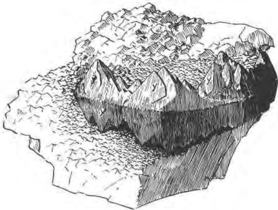
FIG. 3. Type 2, Smithsonite.
