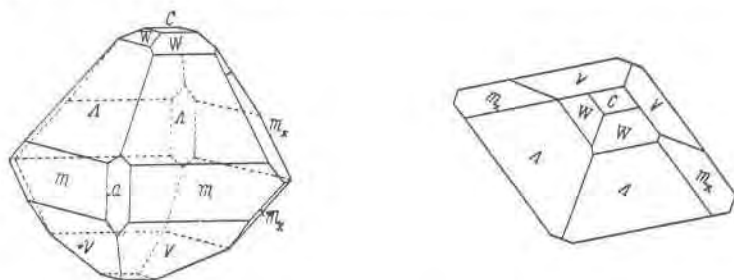
FIG. 3. Datolite
