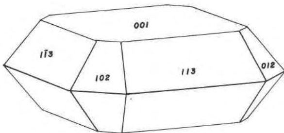
FIG. 1. Avelinoite from the Sapucaia pegmatite mine.
