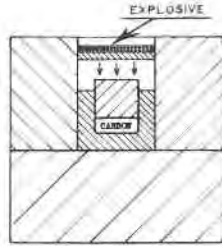
(f) "SHOCK WAVE" APPARATUS
