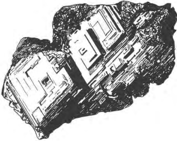
FIG. 8. Gem spessartine.
