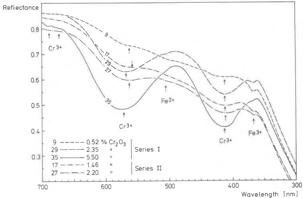
FIG. 2. Reflectance spectra of Stockdale garnets (Amthauer, 1974).
